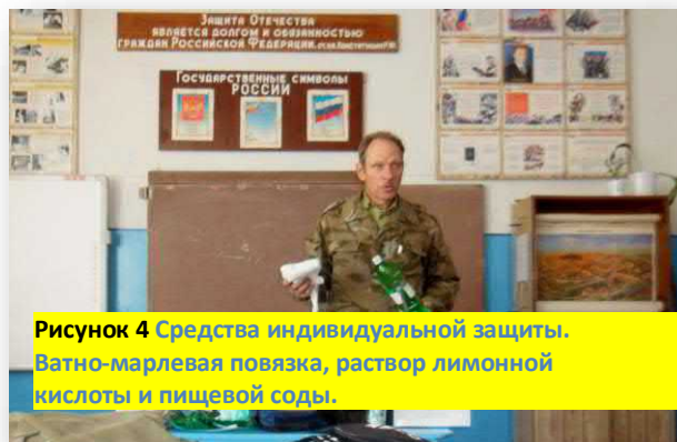
Рисунок 3 Презентация урока
